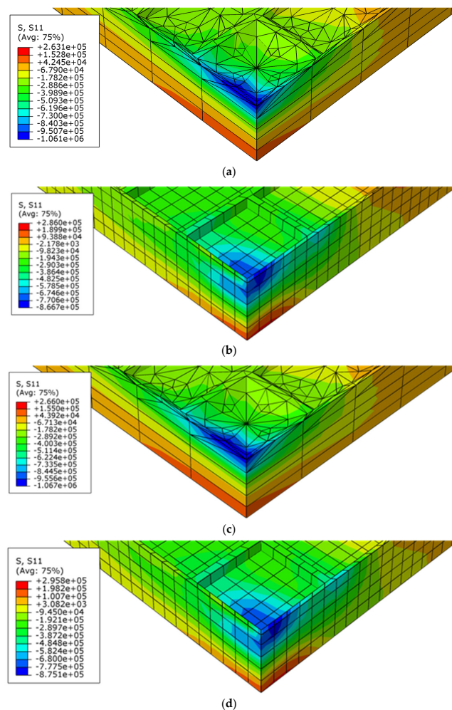
Figure 10. Horizontal stress distribution in the mortar bed: (a) H-SPS + E (subgrade = 180 MPa), (b) R-SPS + E (subgrade = 180 MPa), (c) H-SPS + E (subgrade = 60 MPa), (d) R-SPS + E (subgrade = 60 MPa).
